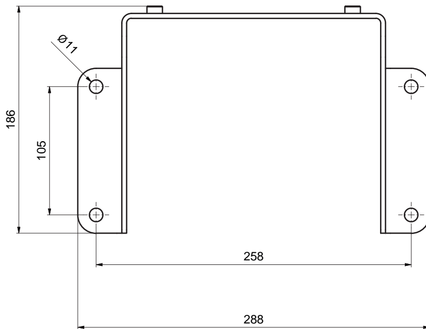
Bild 15.8: Montagewinkel BTF830M
