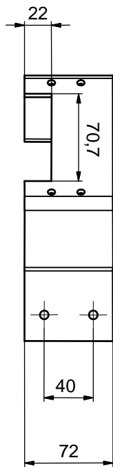
Bild 15.12: Montagewinkel BT856M
