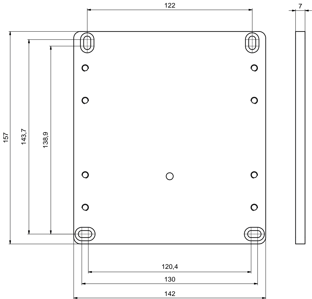
Bild 15.14: Adapterplatte Bohrbild RS4/ROD4 BT800MA
