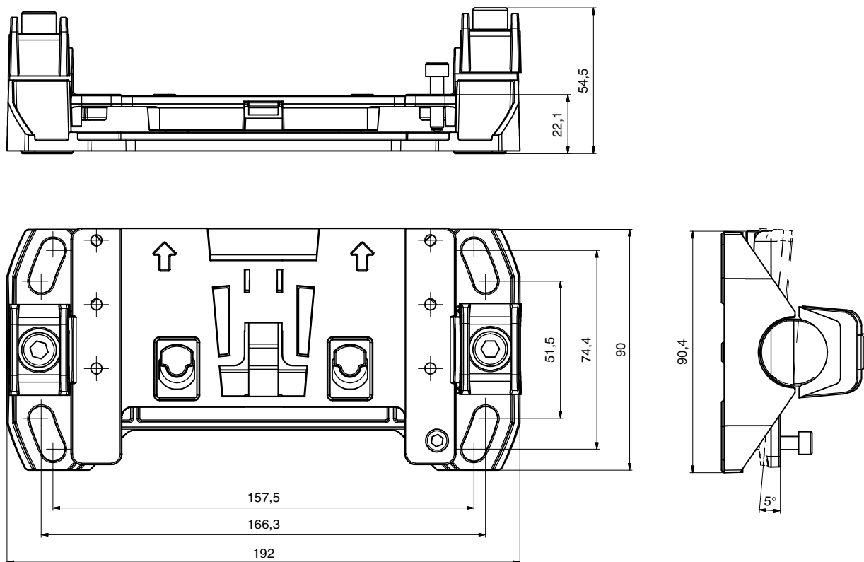
Bild 15.6: Montagesystem BTU800M
