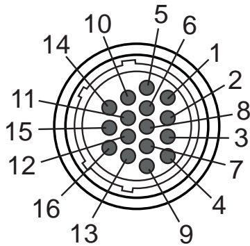
Bild 8.1: Anschlussbelegung M30-Stecker, 16-polig
