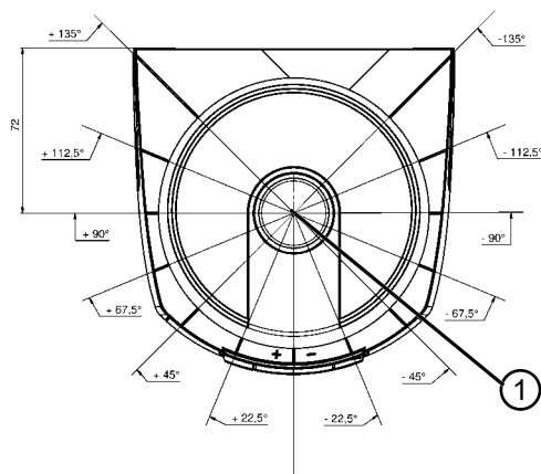
Bild 15.4: Minimaler Platzbedarf zur Montage und zum Austausch der Scannereinheit
