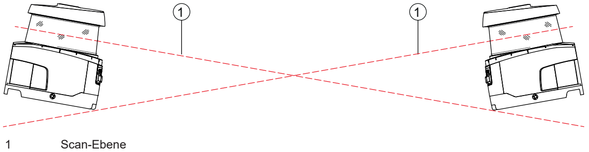
Bild 7.11: Montage gegenüberliegend, ohne Höhenversatz, gekreuzte Ausrichtung
