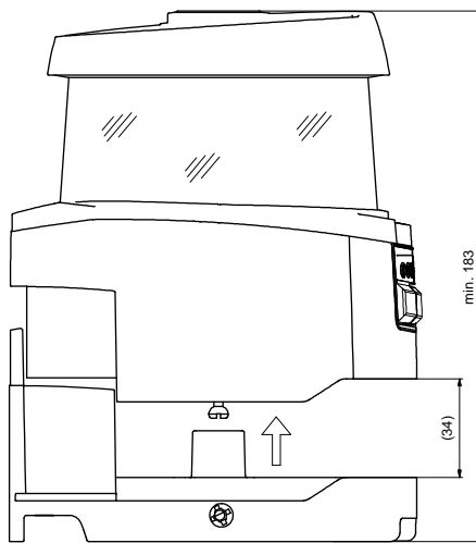
Bild 15.3: Anbaumaße Sicherheits-Laserscanner mit Anschlusseinheit
