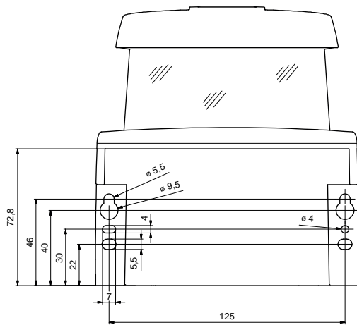
Bild 15.3: Anbaumaße Sicherheits-Laserscanner mit Anschlusseinheit
