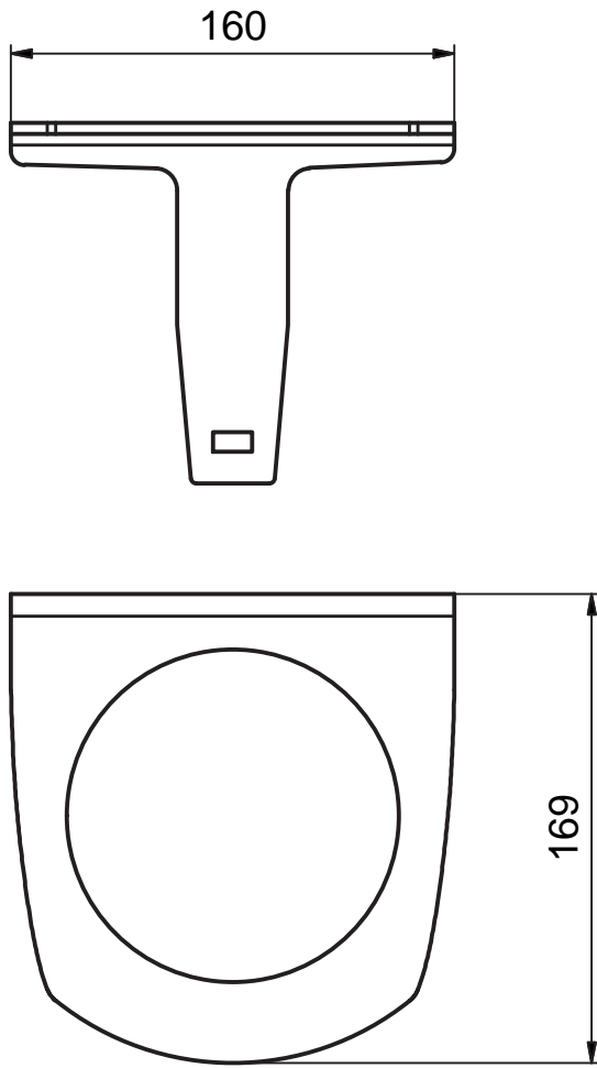
Bild 15.9: Schutzbügel BTP800M
