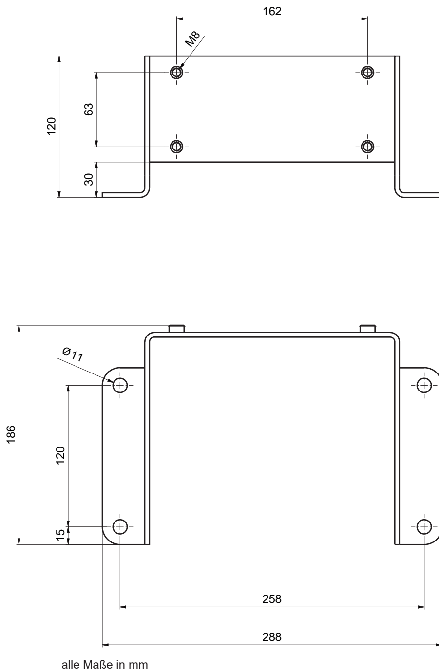
Bild 15.7: Montagewinkel BTF815M
